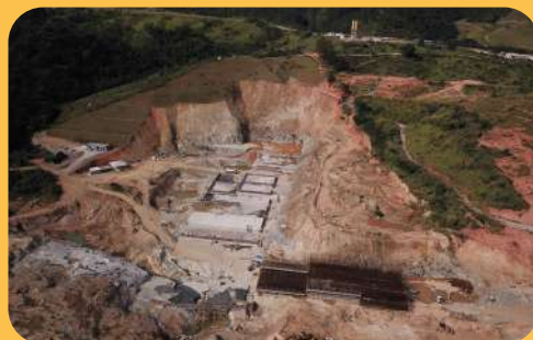
Visão geral da obra. Data: 14/05/22
